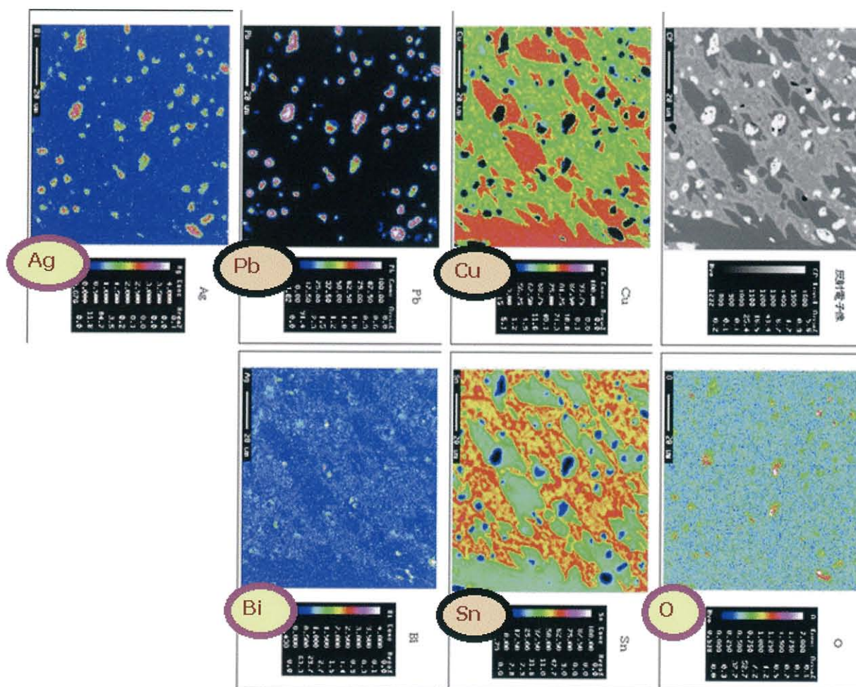
図6 椿井大塚山古墳出土T14鏡の金属組織の元素カラーマッピング
