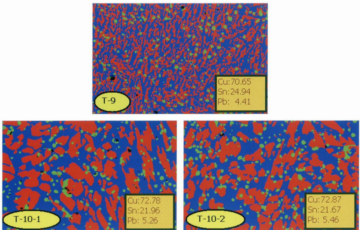
図9 同型鏡（椿井大塚山古墳出土のT9とT10）の金属組織の比較
