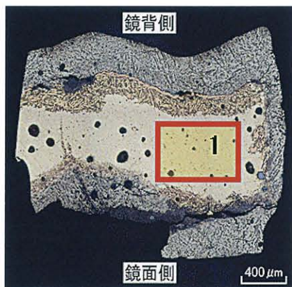
図3 椿井大塚山古墳出土T3鏡の断面観察（光学顕微鏡）
