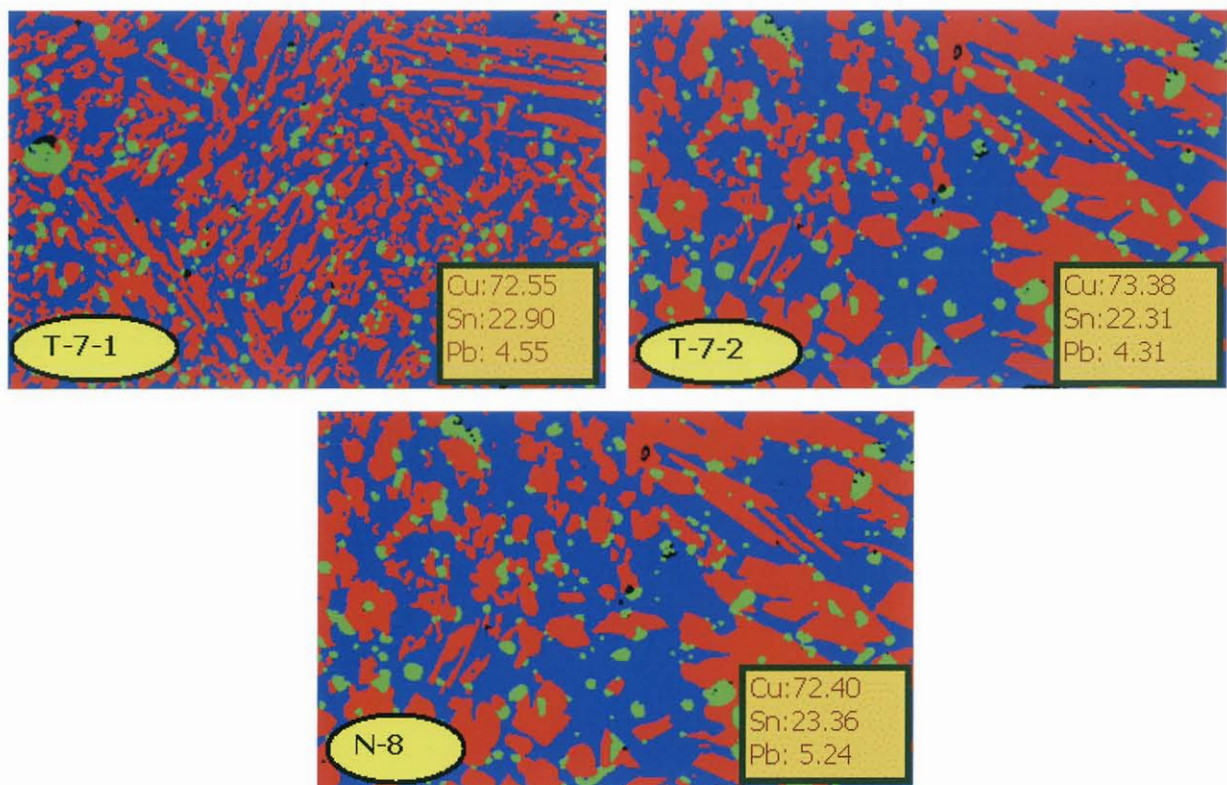
図8 同型鏡（椿井大塚山古墳出土のT7，西求女塚古墳出土のN8）の金属組織の比較
