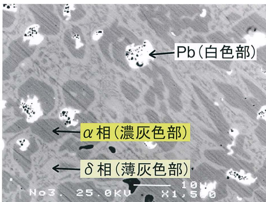
図5 椿井大塚山古墳出土T3鏡の金属組織（SEM観察）
