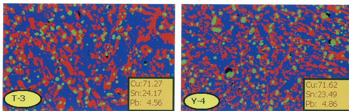
図7 同型鏡（椿井大塚山古墳出土のT3、雪野山古墳出土のY4）の金属組織の比較
