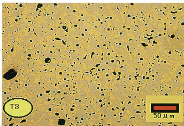
図4 椿井大塚山古墳出土T3鏡の金属組織（光学顕微鏡観察）（図3中の1部分）
